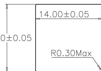
固定板孔尺寸图 T=1.5mm
